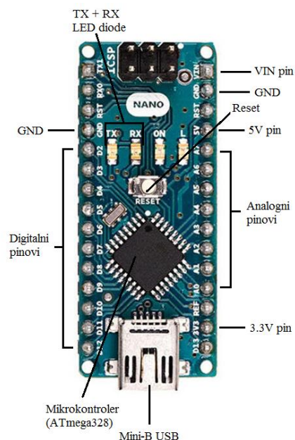
Slika 2.1. Arduino nano pločica [18]
