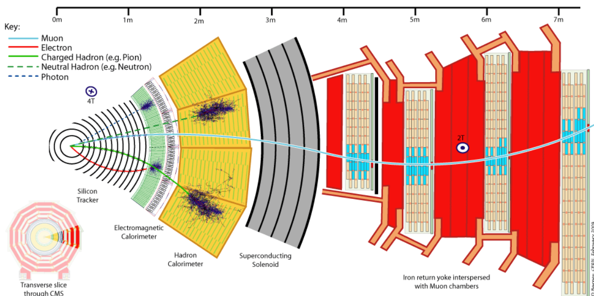
Slika 2.2: Prikaz slojeva CMS detektora
