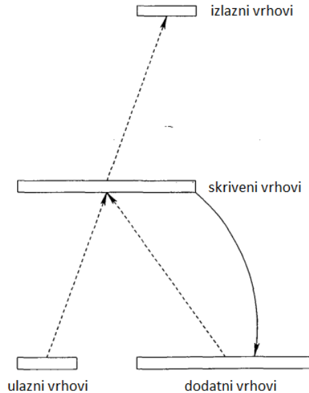
Slika 3.1: Elmanova mreža [1]
