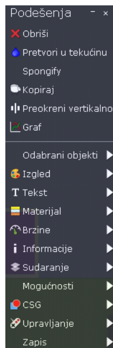
Slika 3.1.7 – Svojstva objekta.
