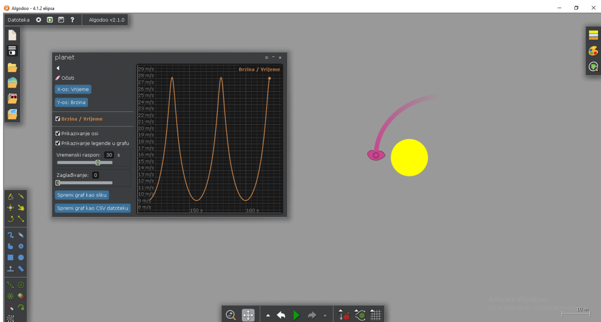
Slika 4.1.3 – Trag crtala kada planet prolazi kroz perihel.
