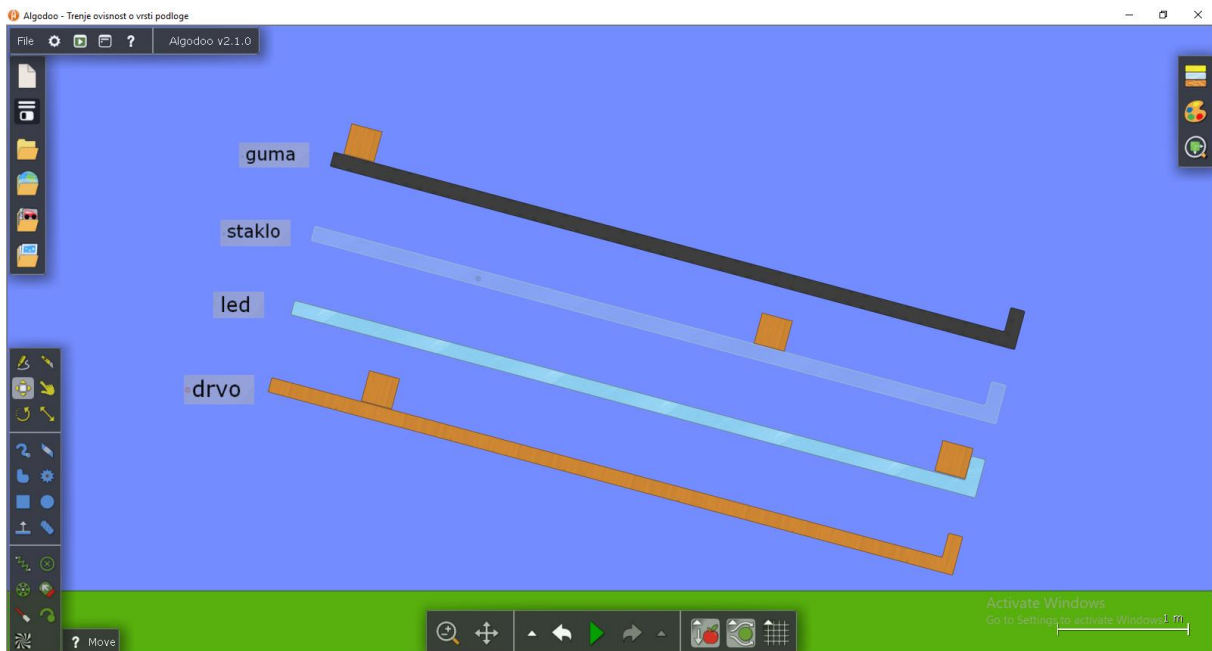
Slika 4.2.14 - Ovisnost trenja o hrapavosti površine.
