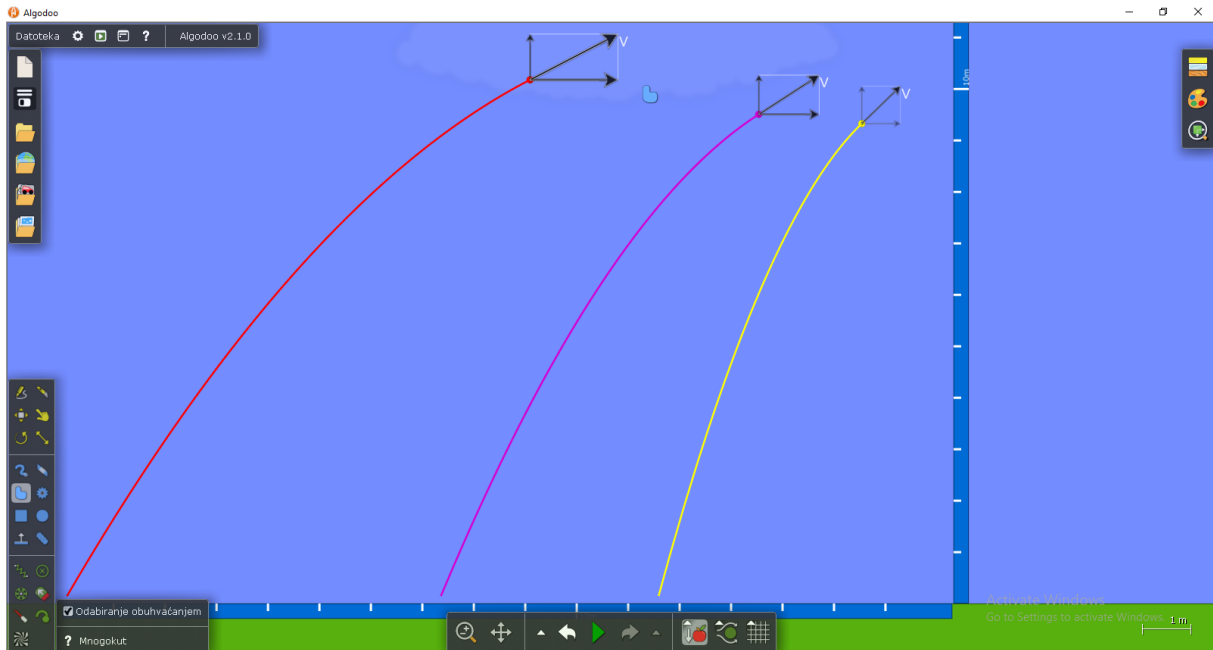
Slika 3.2.2 – Kosi hitac.
