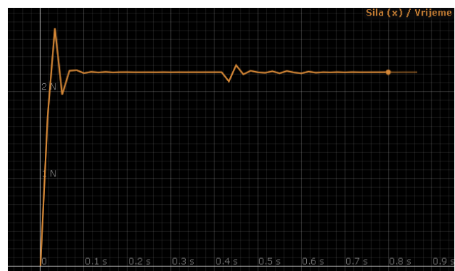
Slika 4.2.9- Graf rezultantne sile za tijelo mase 2 kg.
