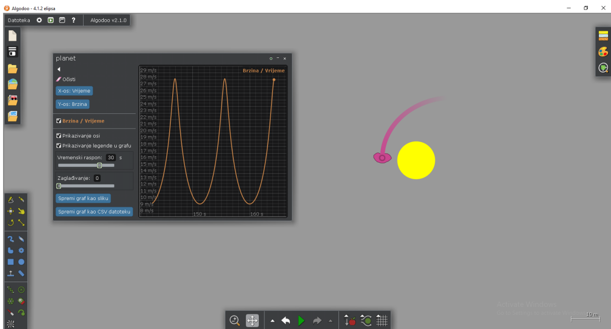
Slika 4.1.5 – Prikaz crtanja grafa brzine planeta u ovisnosti o vremenu.
