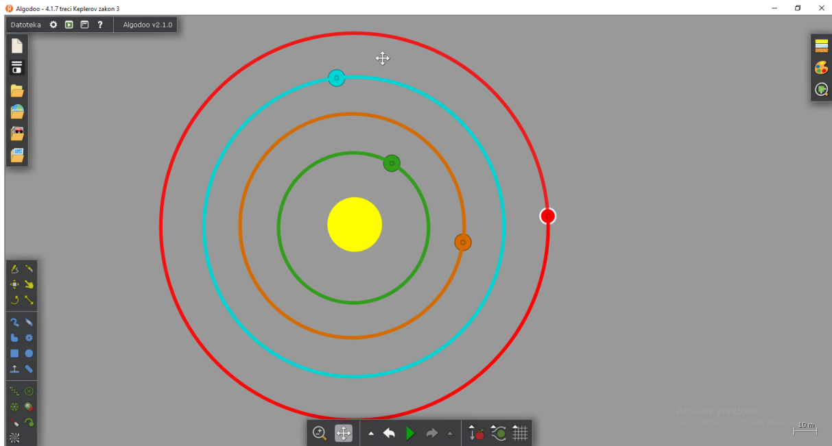
Slika 4.1.7 – Planeti u kružnoj orbiti oko Sunca.
