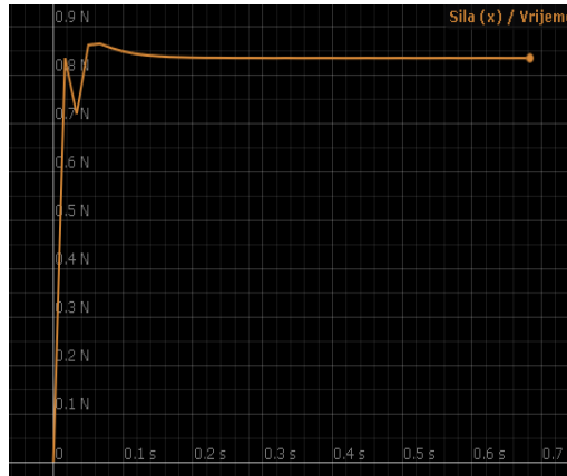
Slika 4.2.10- Graf rezultantne sile za tijelo mase 3 kg.
