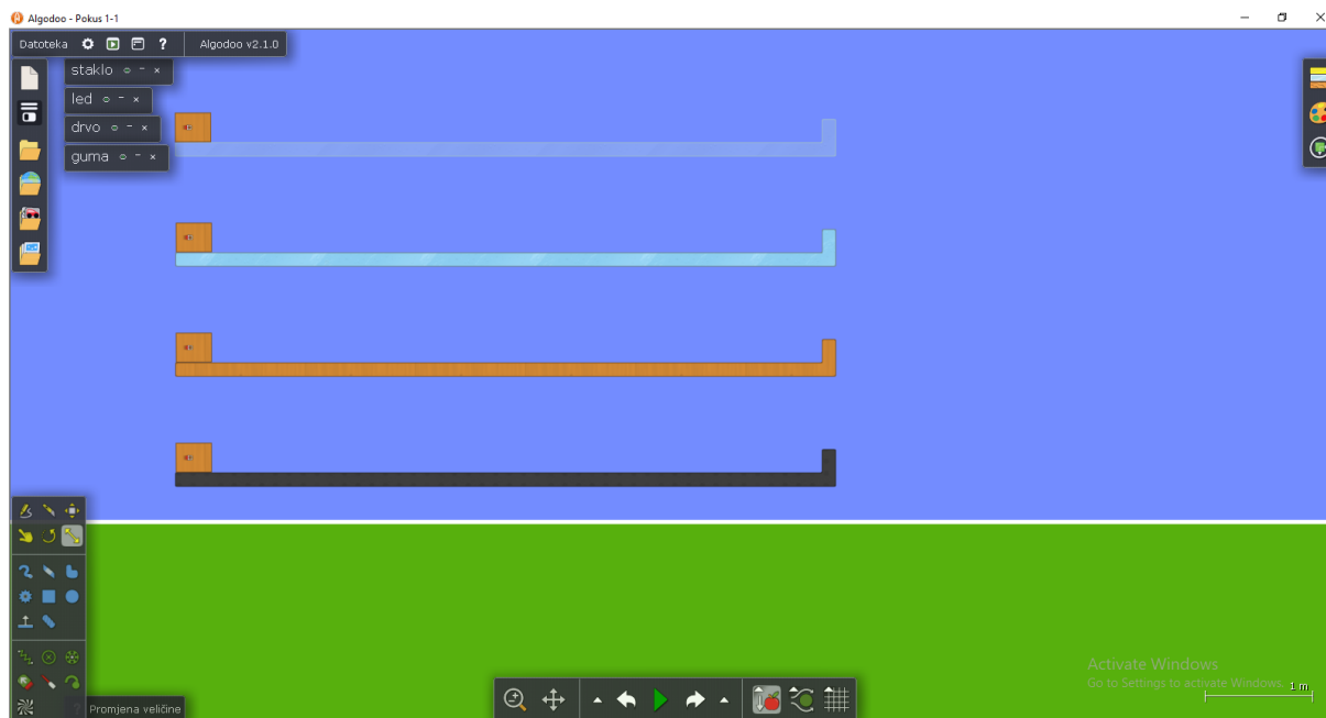
Slika 4.2.1 – Ispitivanje ovisnosti trenja o vrsti površine.
