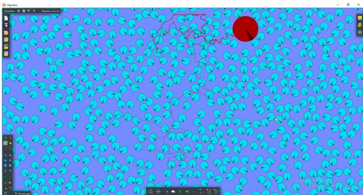
Slika 3.2.3 – Brownovo gibanje.
