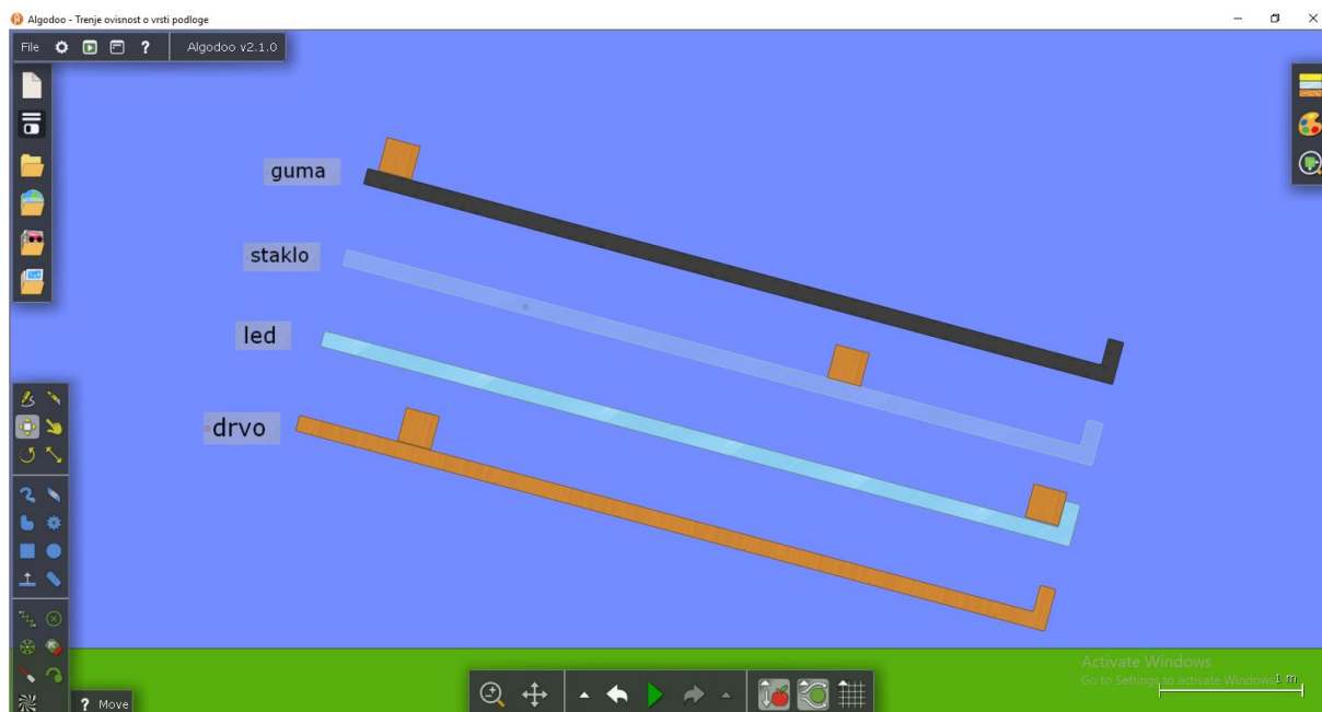
Slika 4.2.14 - Ovisnost trenja o hrapavosti površine.
