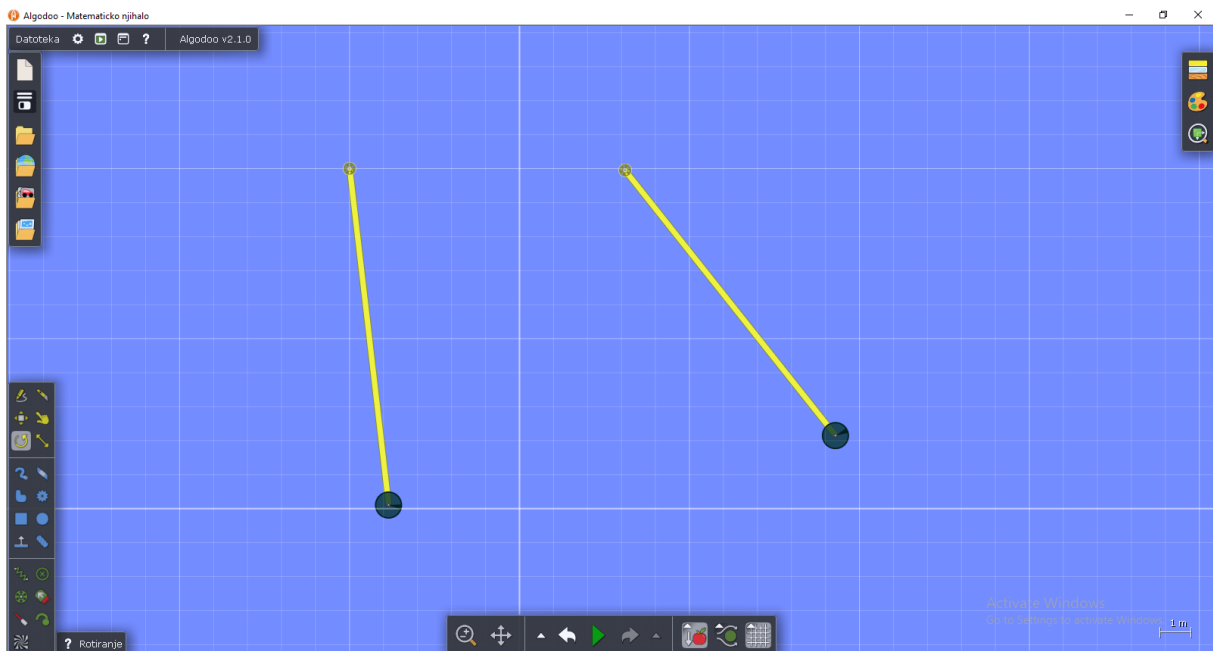
Slika 3.2.13 – Jednaka matematička njihala s različitom amplitudom titranja.
