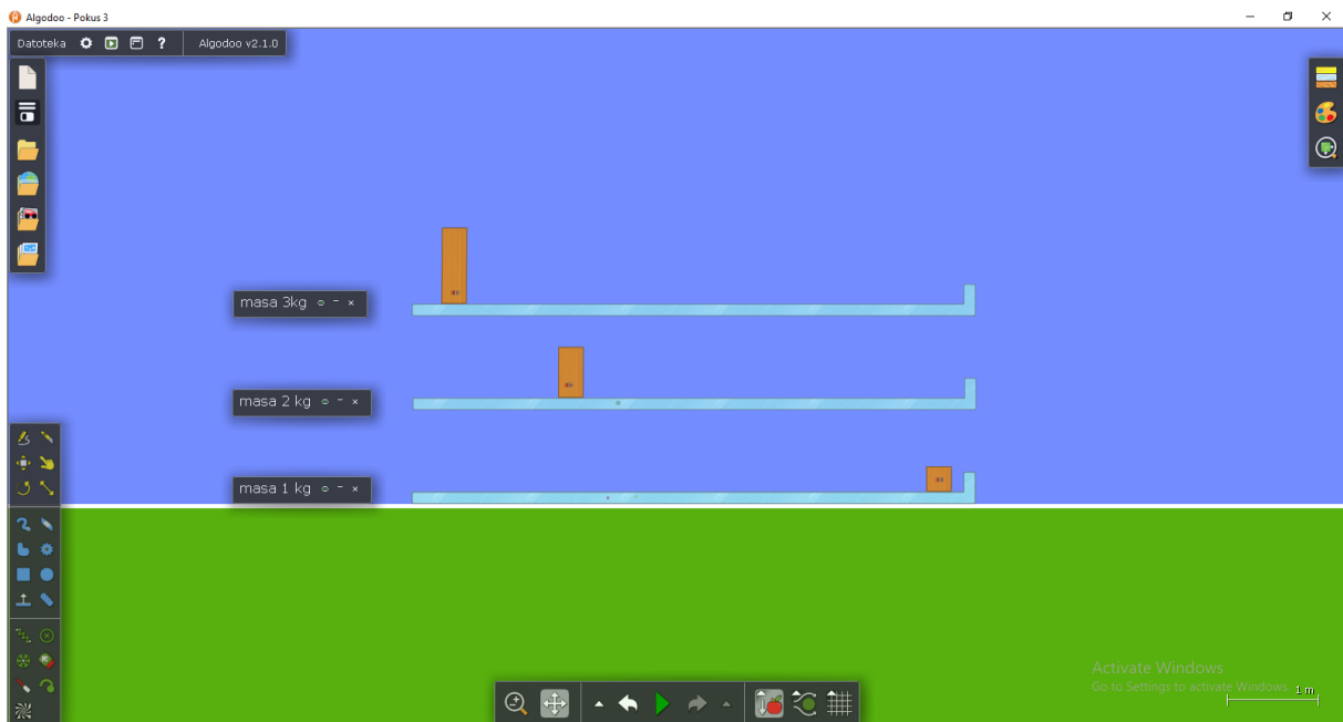
Slika 4.2.6 - Ovisnost trenja o pritisnoj sili – tijekom simulacije.
