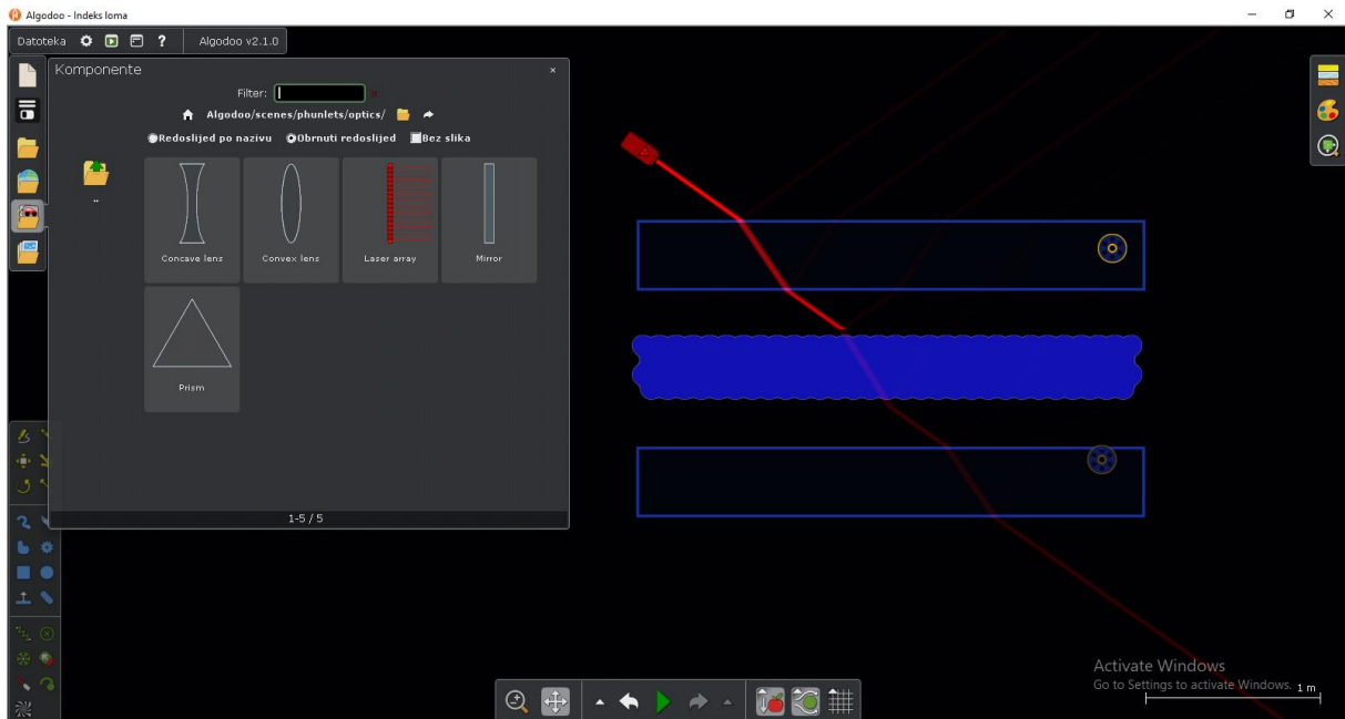
Slika 3.2.9 – Lom crvene svjetlosti kroz dva staklena pravokutnika i vodu između njih.
