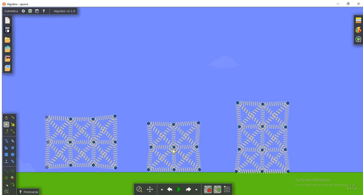
Slika 3.2.17 – Mehanički model spužve.
