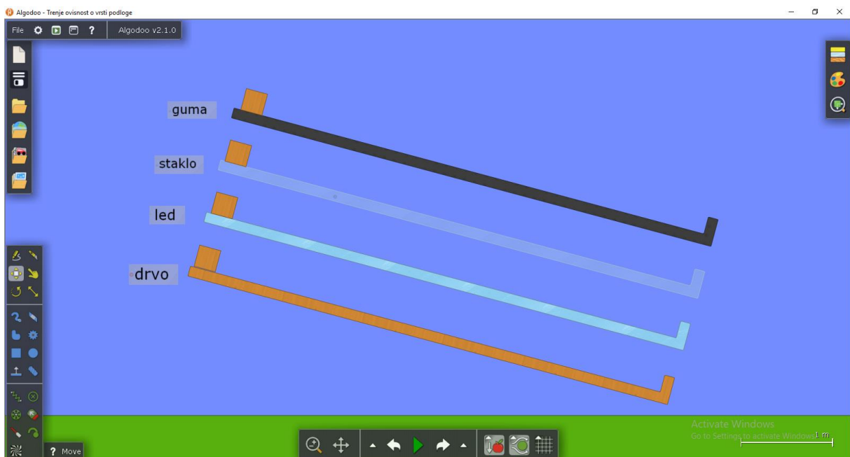
Slika 4.2.13 - Ovisnost trenja o hrapavosti površine.
