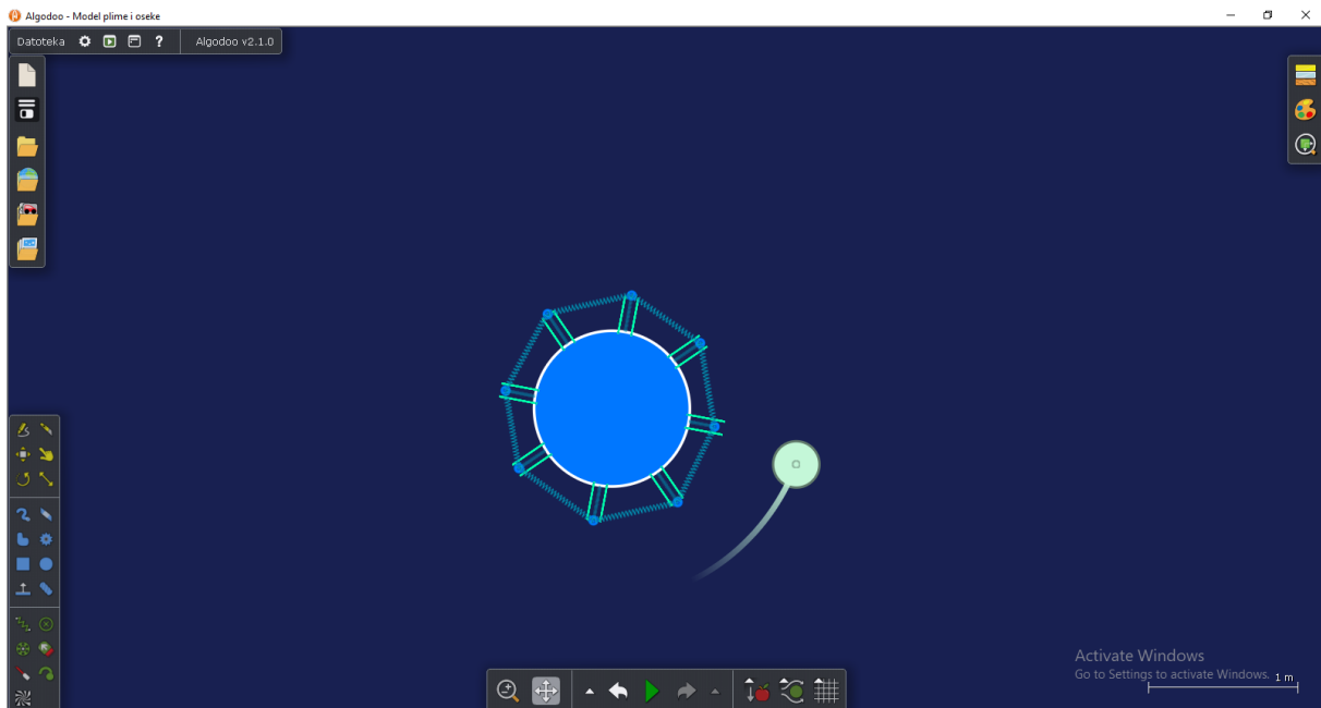
Slika 3.2.11- Model nastanka plime i oseke.
