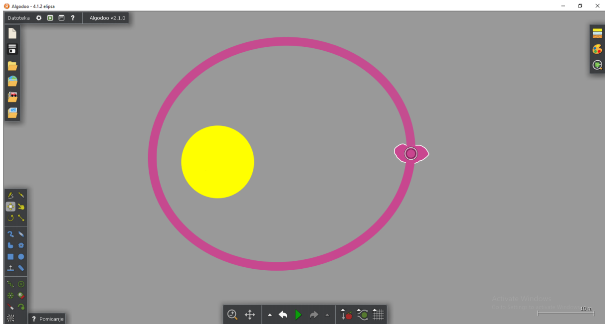
Slika 4.1.2 – Planet u eliptičnoj orbiti oko Sunca.
