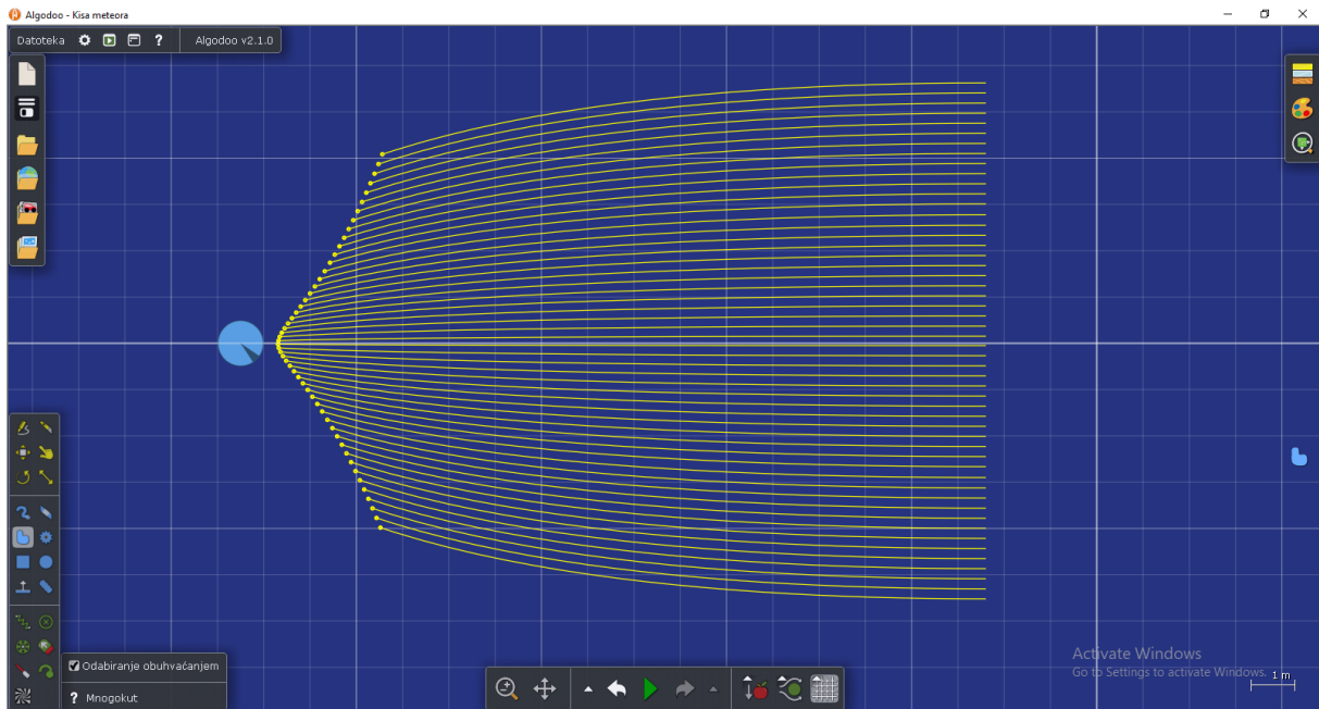
Slika 3.2.12- Simulacija sudara planeta s kišom meteora.
