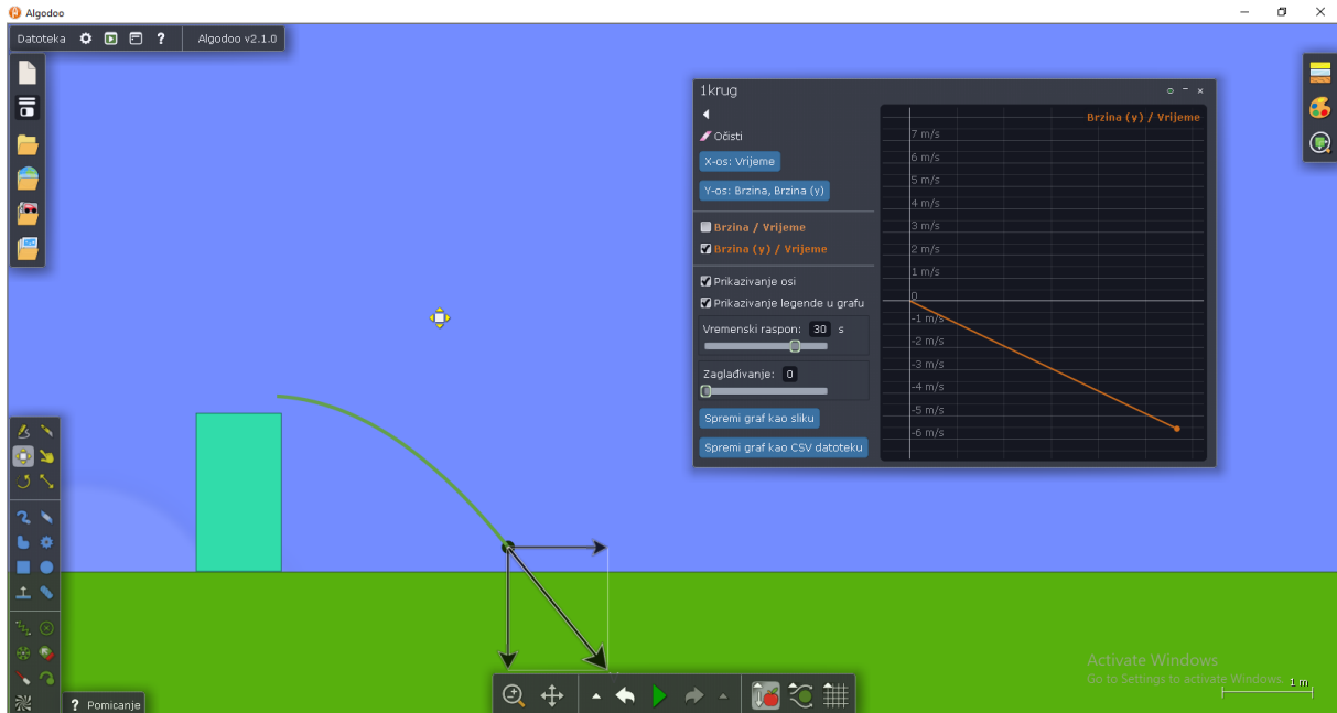
Slika 3.2.16 – Simulacija horizontalnog hitca. Kreirali smo četverokut i na njegov vrh postavili krug. Krugu smo u opcijama dali početnu brzinu u x smjeru te smo uključili prikaz vektora brzine. Dodali smo mu opcijom „crtalo“ trag, a opcijom „graf“ promatramo ovisnost y komponente brzine o vremenu.
