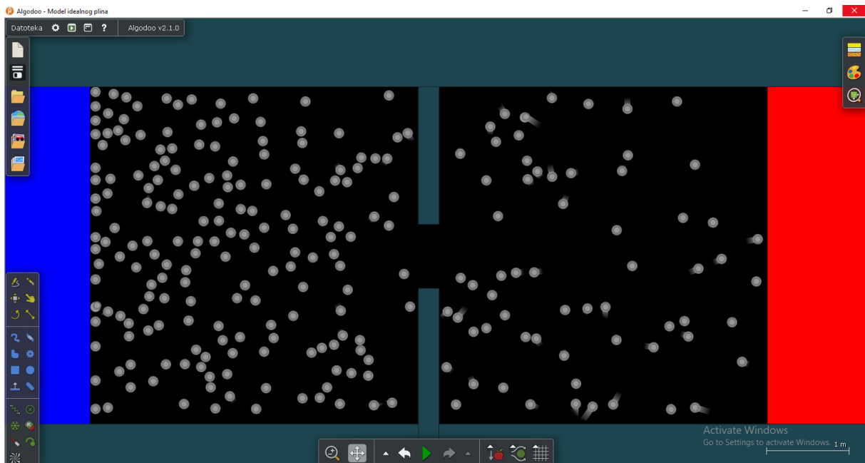
Slika 3.2.10 – Raspodjela čestica idealnog plina u slučaju gradijenta temperature.
