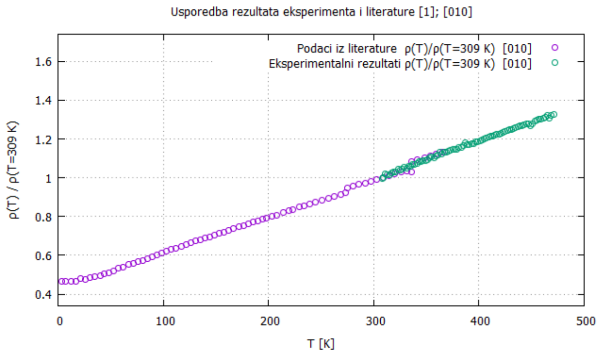
Slika 25. Ovisnost električne otpornosti o temperaturi duž kristalografske orijentacije [010].
