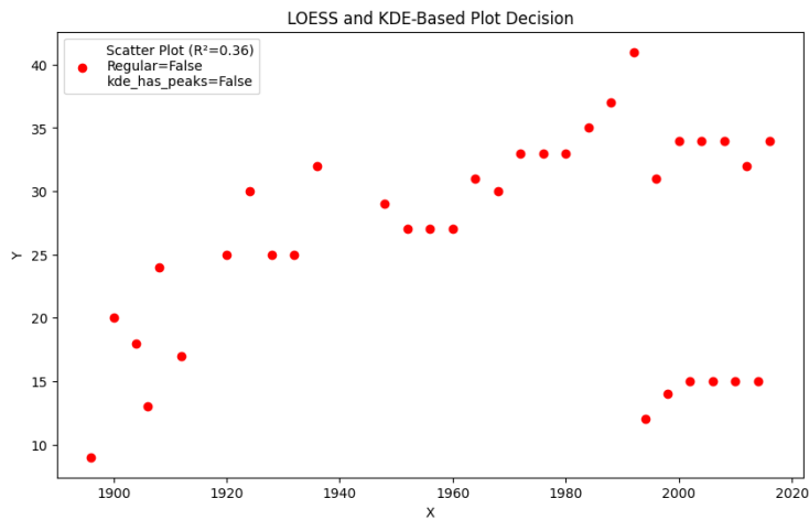
Slika 32 Raspršeni dijagram
