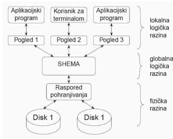
Sl. 1.1 Arhitektura baze podataka
