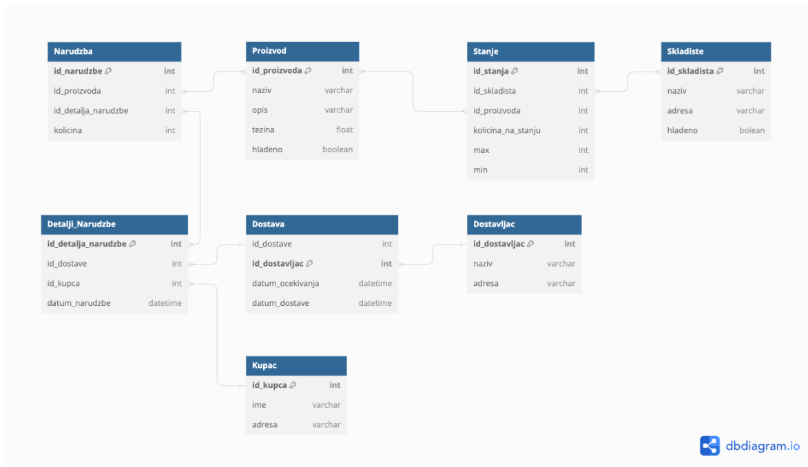
Slika 4.1 - ERD Dijagram
