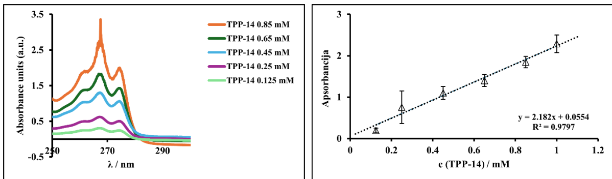
Apsorpcijski spektar i baždarna krivulja spoja TPP-14
