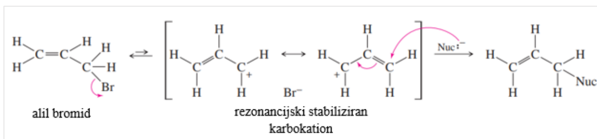
Slika 9. Rezonancijska stabilizacija alil bromida (izvor: Wade, 2013)
