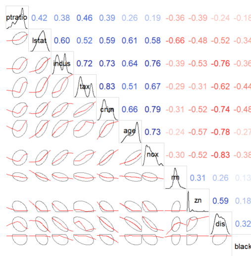
Slika 4.1: Prediktori grupirani prema korelaciji.
