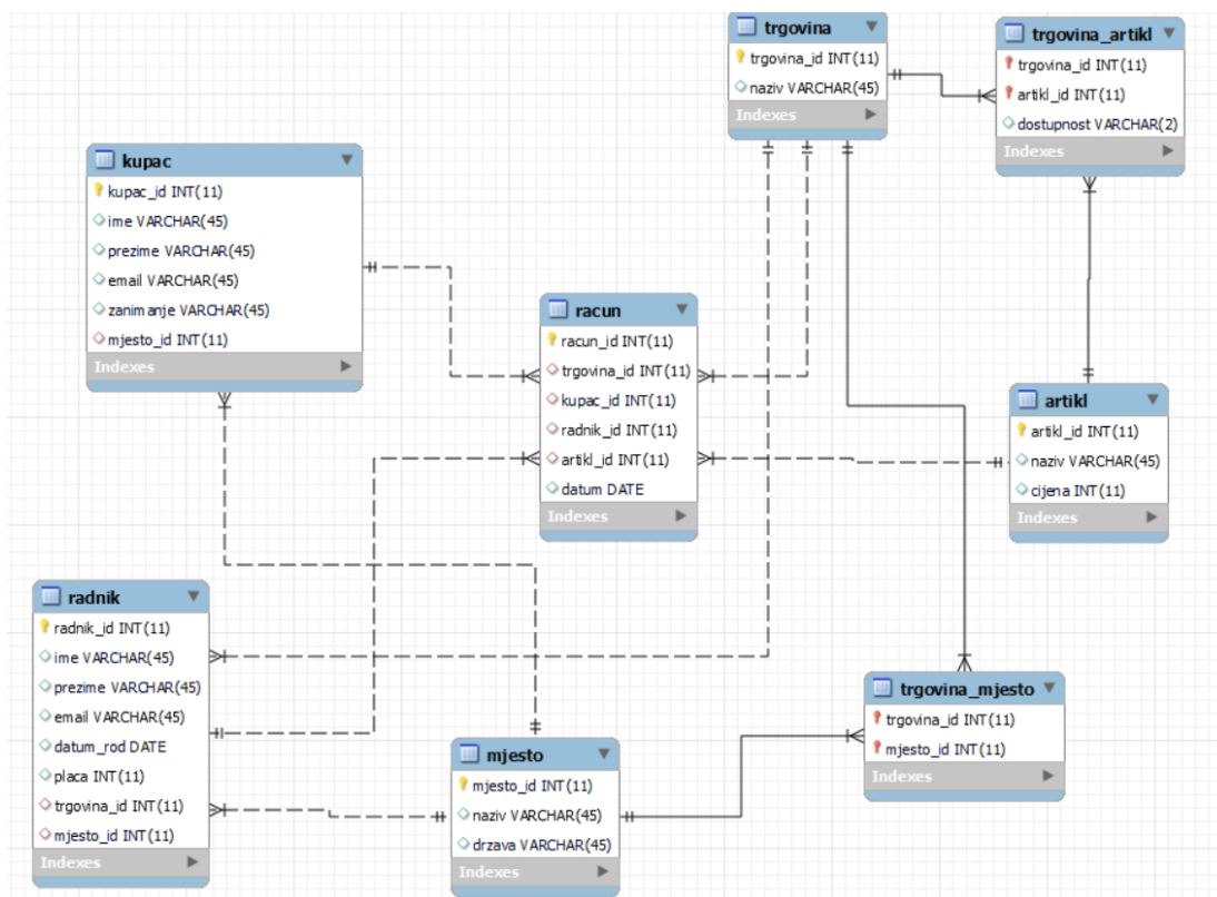
Slika 5 Dijagram baze podataka MySQL
