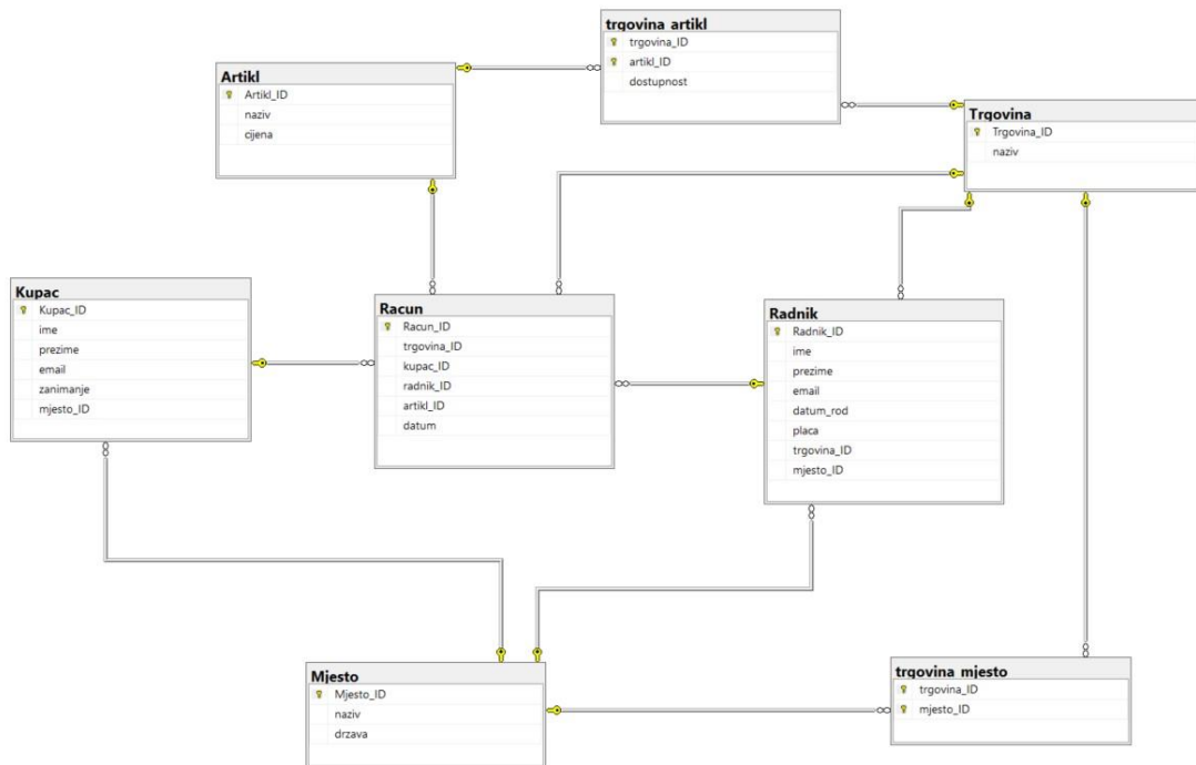
Slika 4 Dijagram MSSQL
