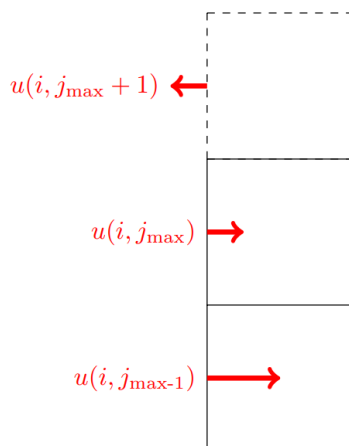
Slika 6: Prikaz postavljanja Dirichletovog rubnog uvjeta za u brzinu na gornjoj stijenci domene. Vrijednost u u fiktivnoj ćeliji ( j_{max} + 1 ) postavljamo na suprotnu vrijednost od ćelije ispod ( j_{max} ) kako bi između njih (na rubu domene) vrijednost bila 0. (Slika preuzeta iz [6])
