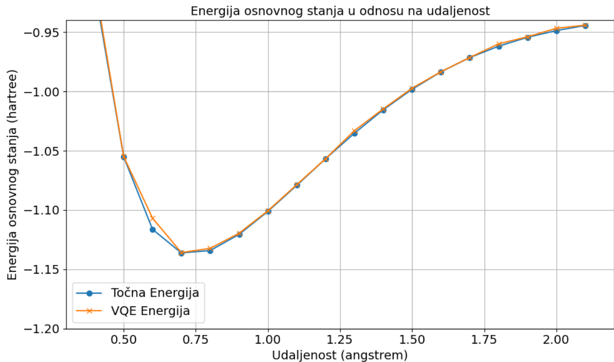
Slika 24: Graf prikazuje ovisnost energije osnovnog stanja molekule H_2 o udaljenostima među atomima vodika u molekuli. Također je prikazana i energija dobivene klasičnom metodom koju koristimo kao referentnu vrijednost. Simulacija je izvršena na idealnom kvantnom računalu. Korišten je COBYLA optimizator.
