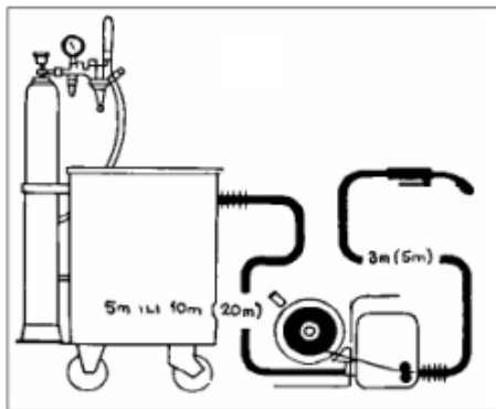
Slika 9: Univerzalni sustav za dovodjenje žice[12]
