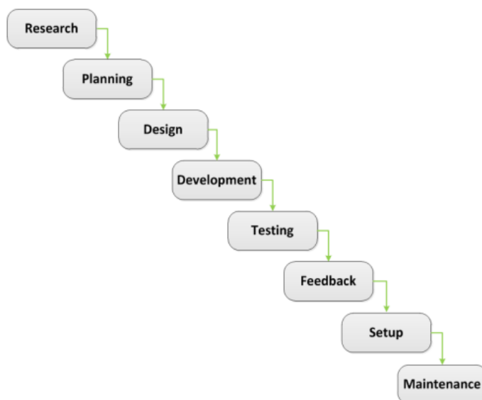
Slika 1.1 Model Vodopada [3]
