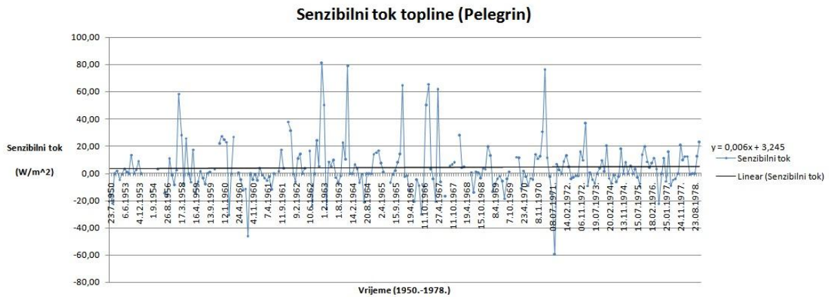
Slika 2.4. Senzibilni tok topline i trend
