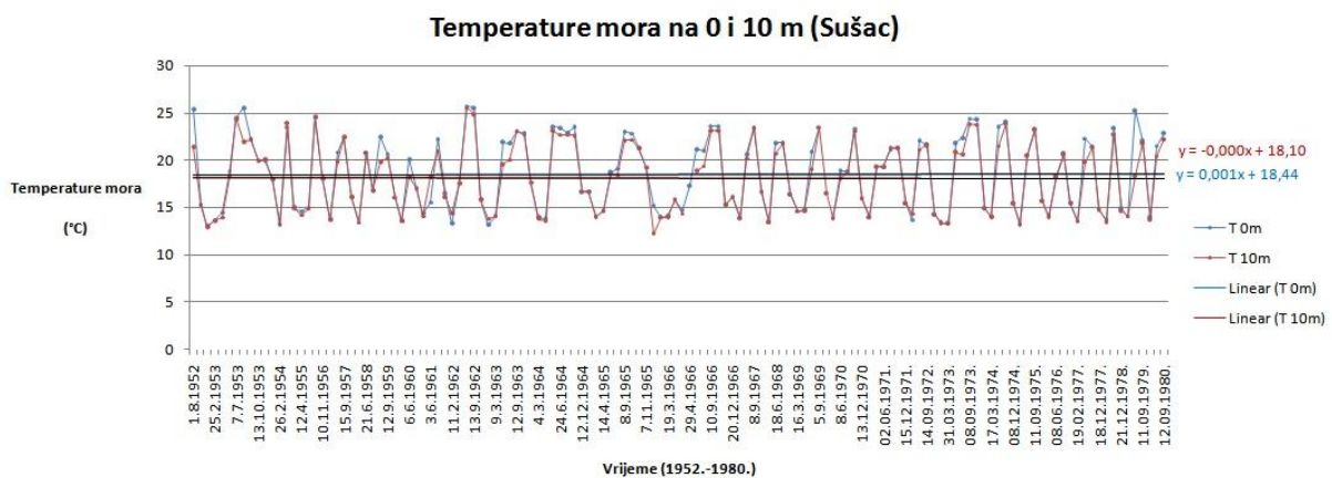
Slika. 2.11. Temperature mora i trendovi
