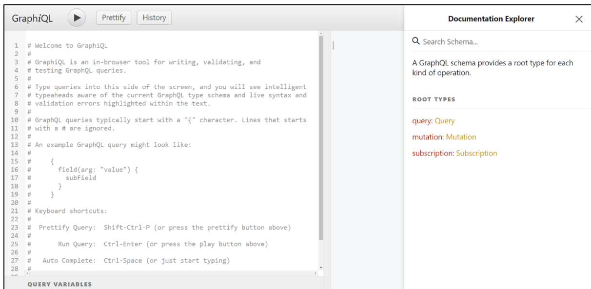
Slika 14 - GraphiQL
