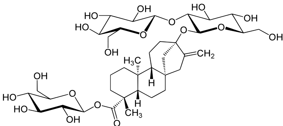
Slika 2. Molekula steviozida
