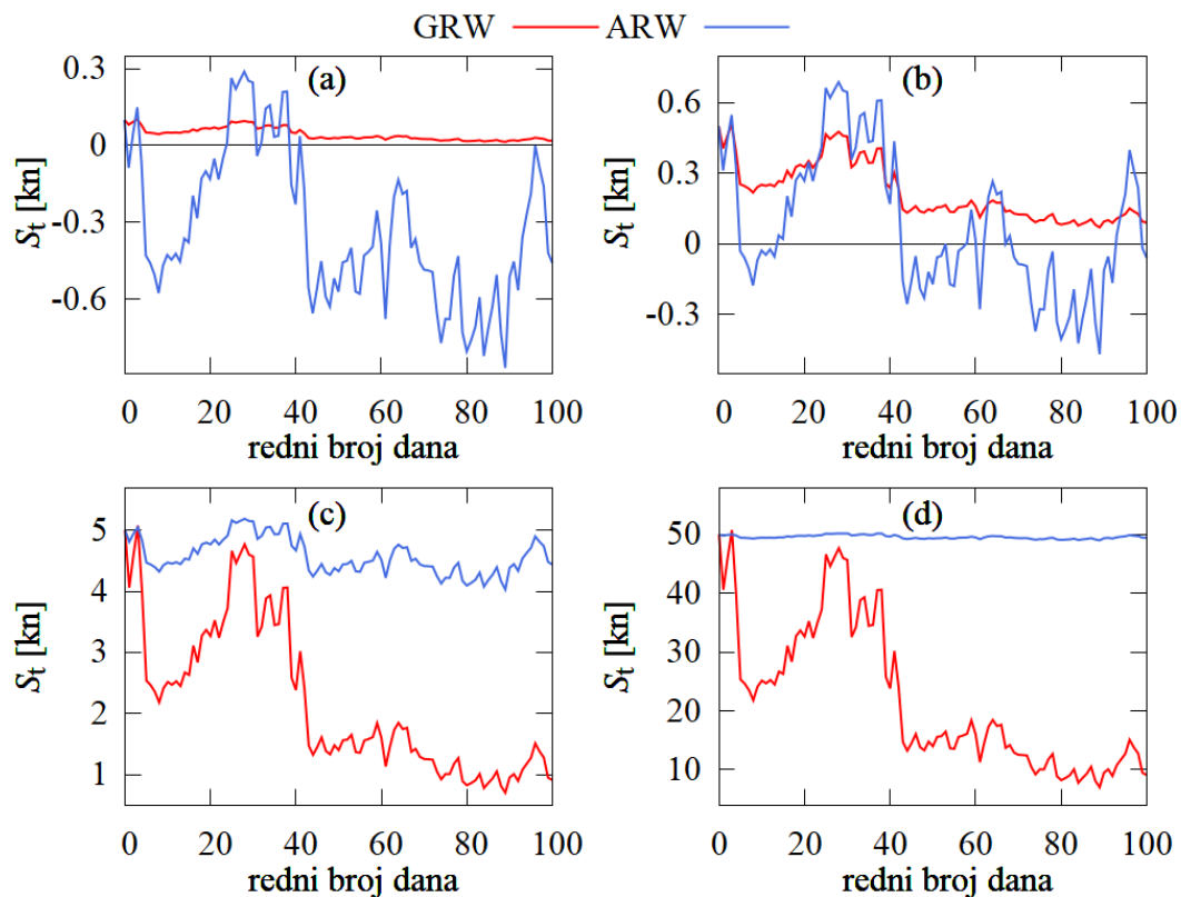
Crtež 4: Usporedba geometrijskog i aritmetičkog slučajnog hoda na skali od 100 dana s parametrima \sigma = 300\% , \mu = 0,1 , te ulazom za funkciju ran1 idum = -2. Korištene su različite početne cijene: (a) S_0 = 0,1 kn, (b) S_0 = 0,5 kn, (c) S_0 = 5 kn, (d) S_0 = 50 kn
