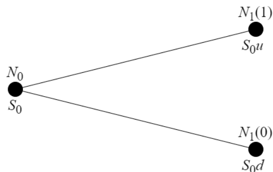
Crtež 8: Prvi korak binomnog stabla
