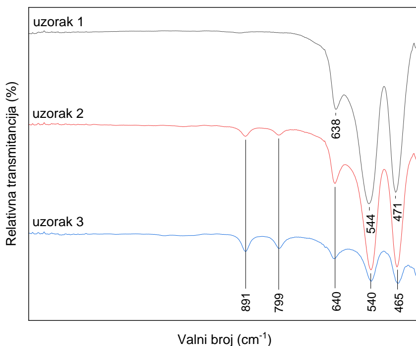
Slika 10. FTIR spektri uzoraka 1, 2 i 3
