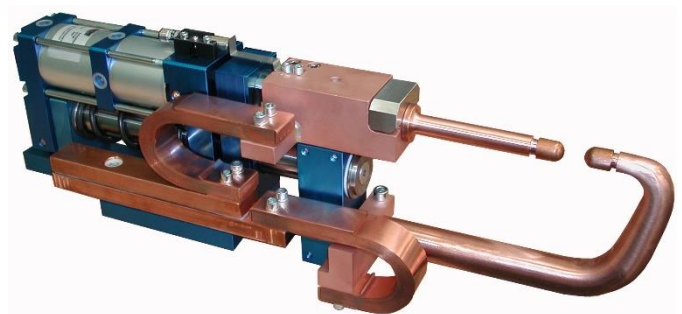
Slika 5.5. C-tip kliješta [21]
