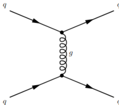
Slika 2: Prikaz QCD procesa preko Feynmannovog dijagrama. Prikazani dijagram interpretiramo na način da vrijeme ide s lijeva na desno. Drugim riječima, lijevo je početno stanje, a desno konačno. q nam je oznaka za kvark, a g za gluon. Slika preuzeta iz [3].
