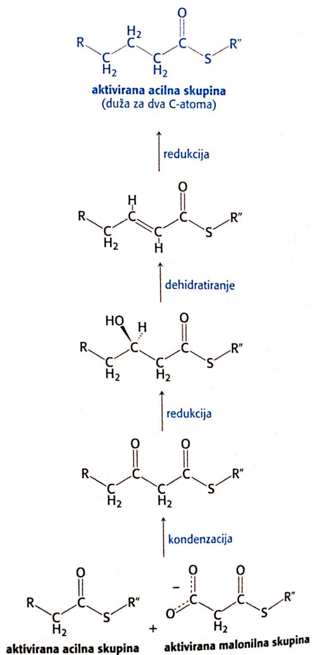
Slika 8. Koraci u razgradnji i sintezi masnih kiselina
