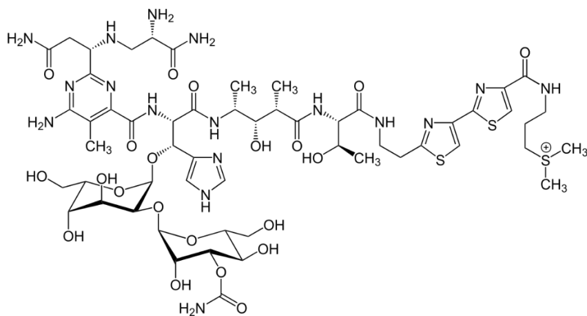
Slika 11. Struktura bleomicina (preuzeto sa https://en.wikipedia.org/wiki/Bleomycin )
