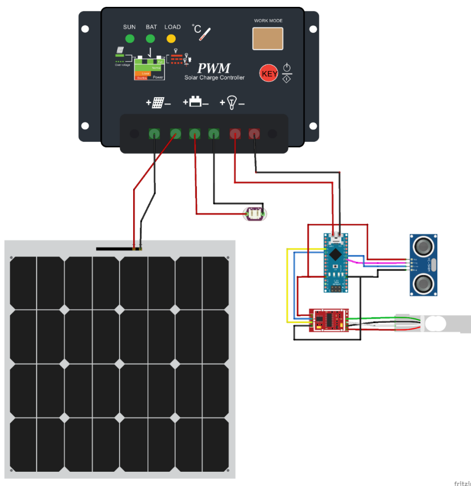
Slika 6.8. Shema spoja svih komponenti projekta sa Arduino
