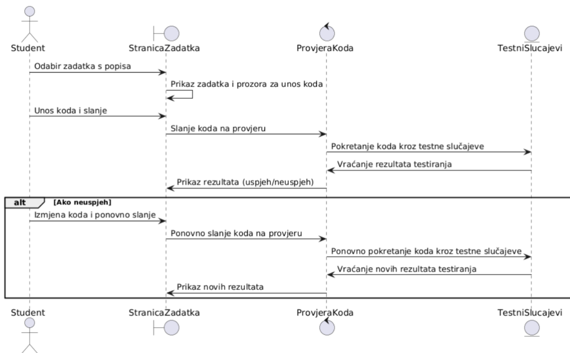
Slika 8 Dijagram slijeda
