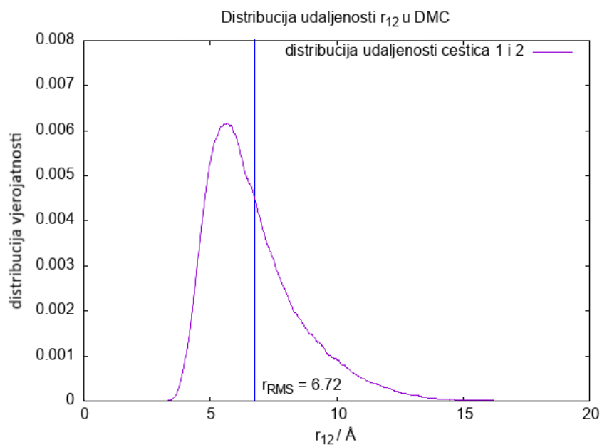
Slika 25: Distribucija udaljenosti r_{12} između čestica šetača
