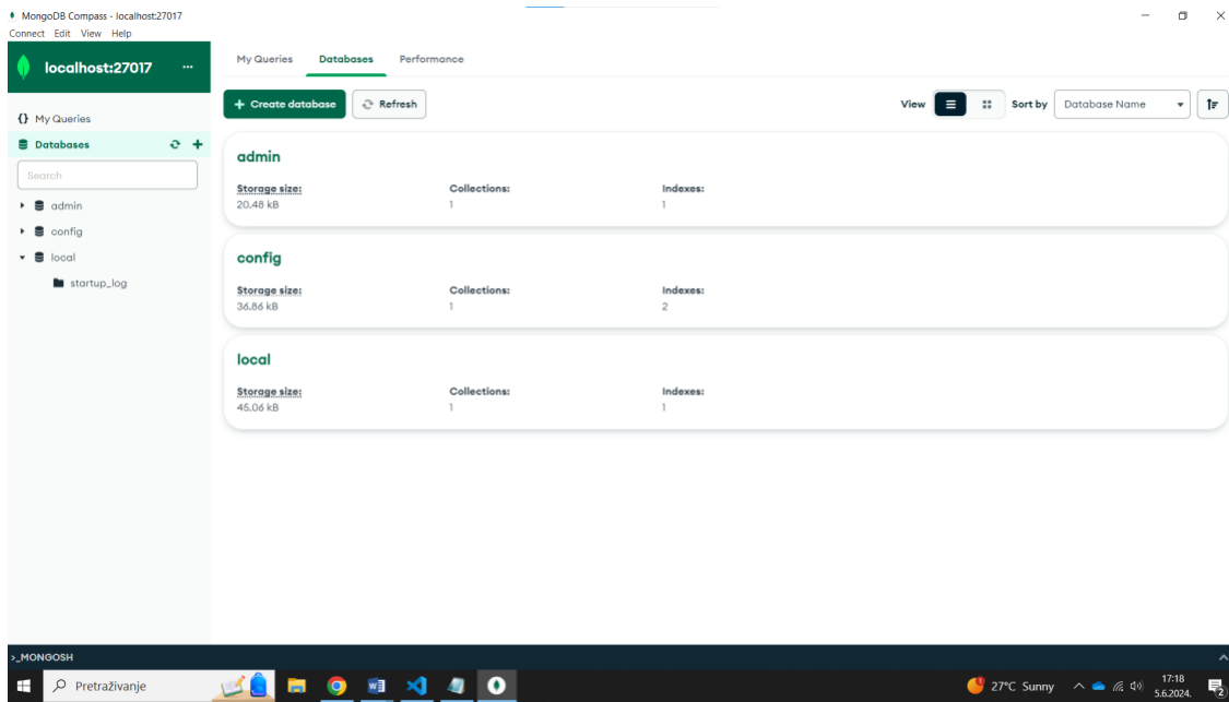
Slika 3. Sadržaj MongoDB
