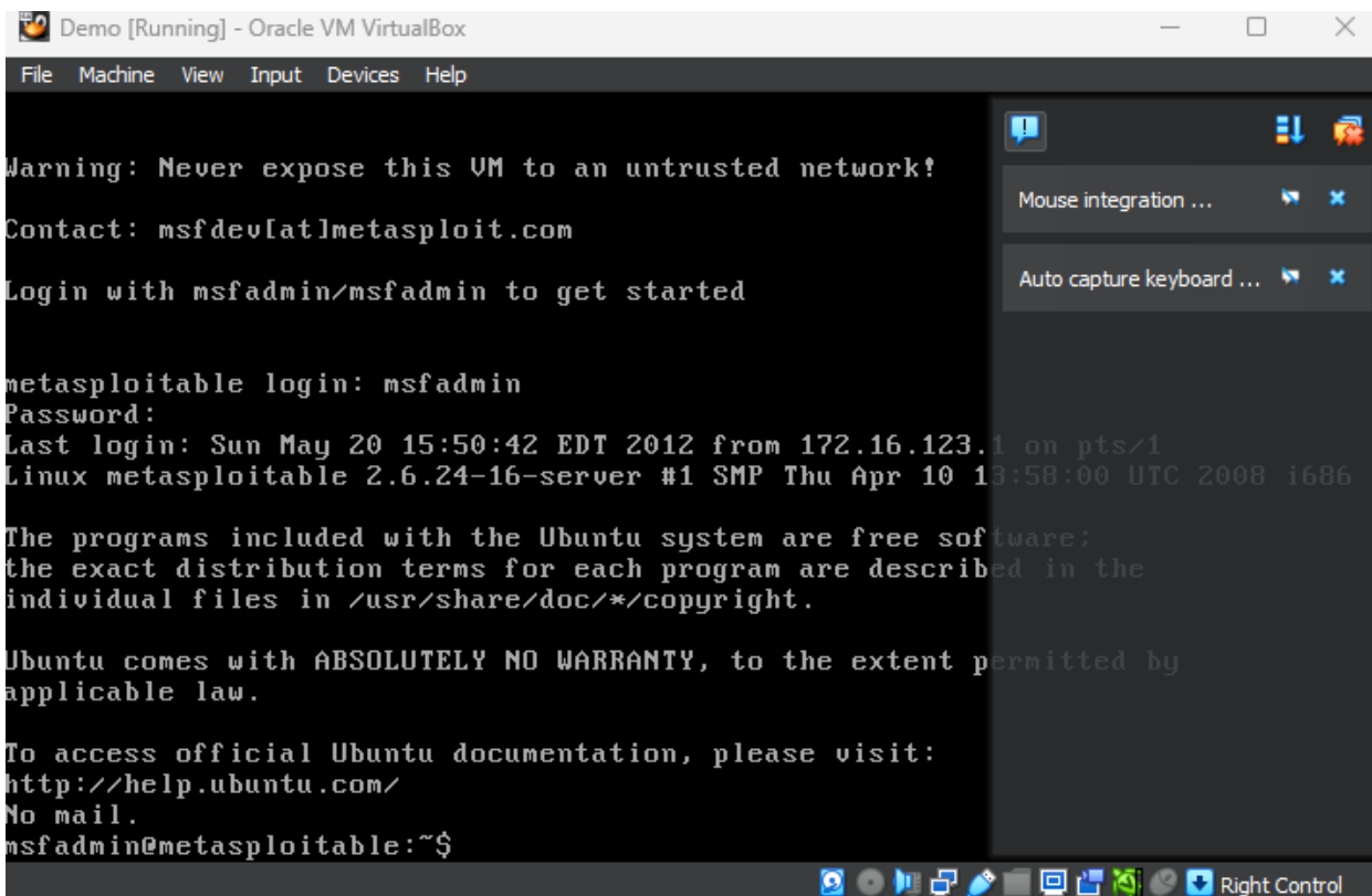
Slika 2.12 Metasploitable Linux
