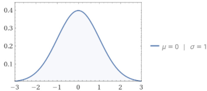
Slika 1.1: Gaussova krivulja
