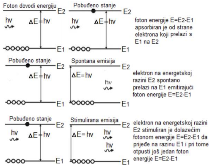
Slika 3.2 Ukratko objašnjen proces nastanka laserske svjetlosti (slika preuzeta s http://repositorij.fsb.hr/5112/1/Antoli%202016_Zavr%20Prediplomski.pdf [10])
