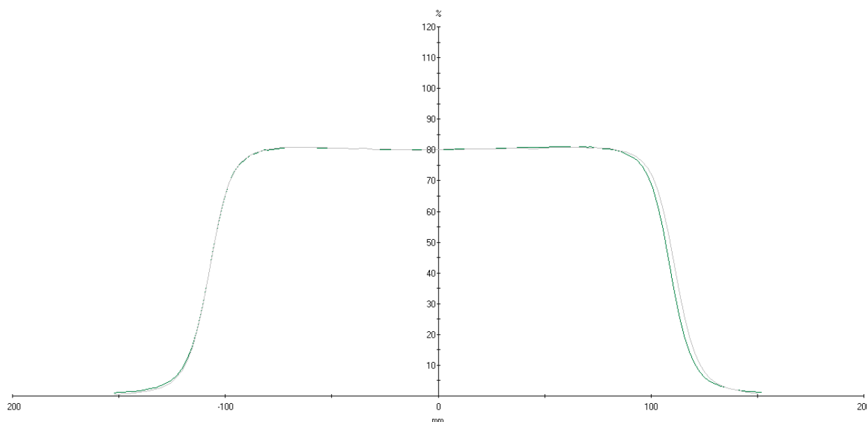
Slika 40. Profili elektronskih snopova energije 16 MeV. Plava krivulja na slici predstavlja „inplane“ profil, a ljubičasta krivulja predstavlja „crossplane“ profil. Na x-osi označena je udaljenost od središnje osi izražena u milimetrima, a na y-osi je označena doza u postotcima. Veličina polja je 20 cm x 20 cm, a SSD je 100 cm.
