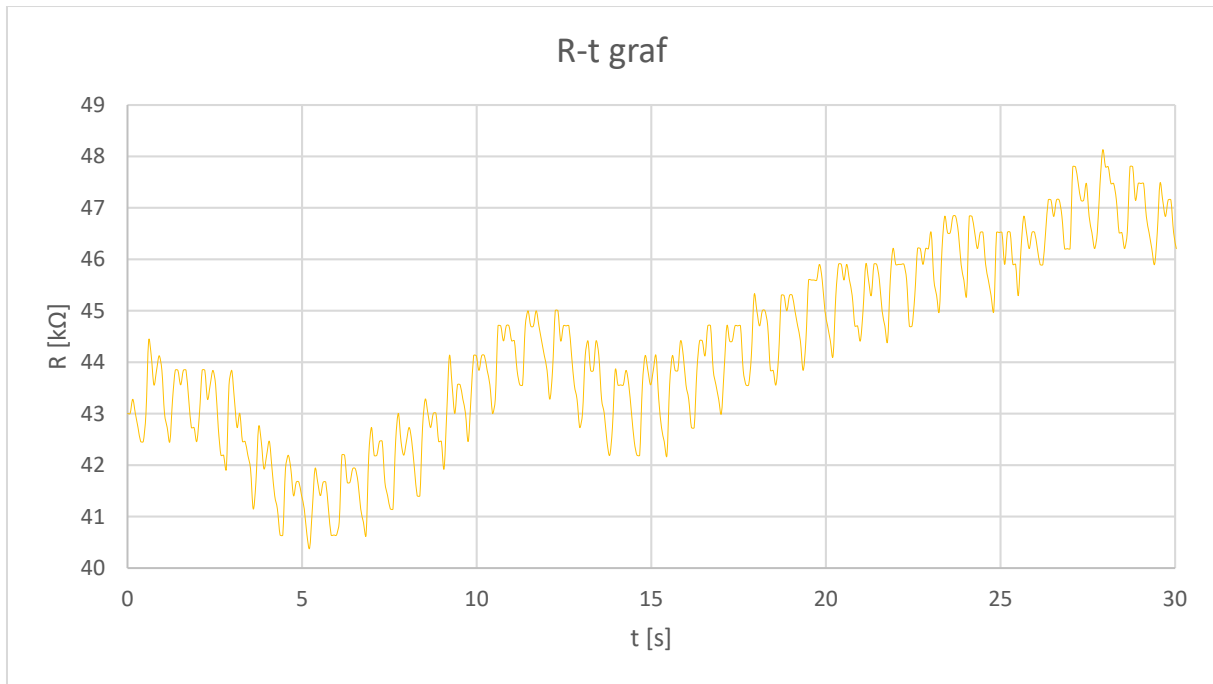
Graf 4. Krivulja kucanja ljudskog srca izmjerena eksperimentalnim uređajem s izvorom svjetlosti žute diode. Graf pokazuje ovisnost otpora na fotootporniku (y-os) o proteklom vremenu (x-os). Unutar 30 sekundi mjerenja srce je napravilo 38 otkucaja s brzinom kucanja 76 otkucaja u minuti.
