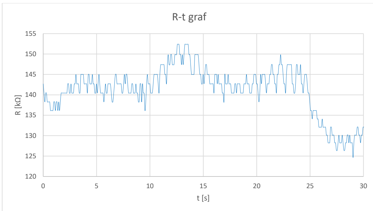
Graf 6. Krivulja kucanja ljudskog srca izmjerena eksperimentalnim uređajem s izvorom svjetlosti plave diode. Graf pokazuje ovisnost otpora na fotootporniku (y-os) o proteklom vremenu (x-os). Unutar 30 sekundi mjerenja srce je napravilo 35 otkucaja s brzinom kucanja 70 otkucaja u minuti.
