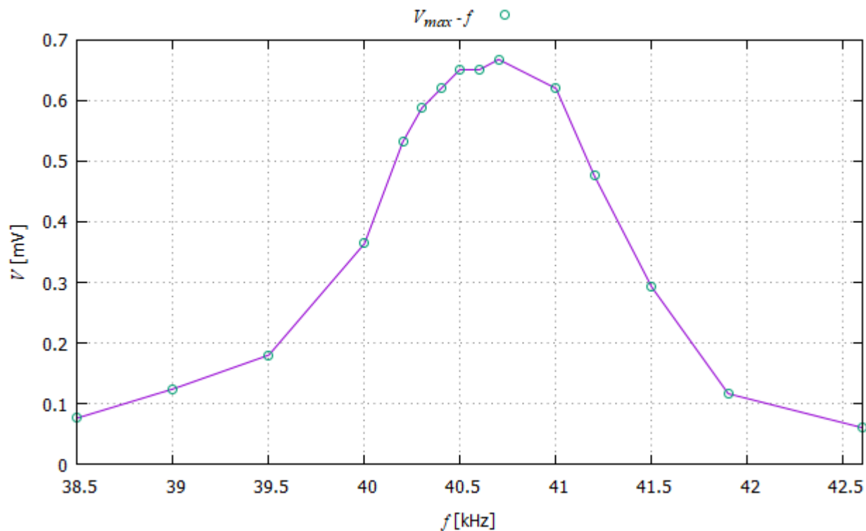
Slika 15: Ovisnost maksimalnog izmjenog napona na prijemniku o frekvenciji upadnog vala.
