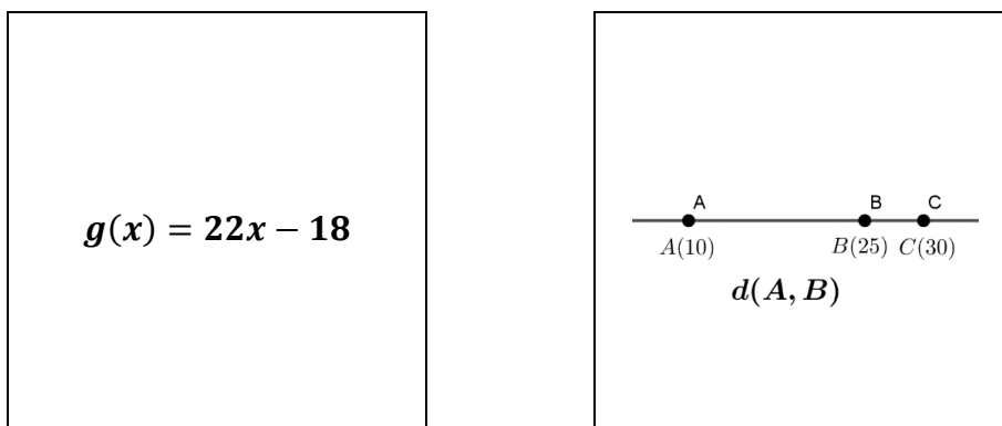
Slika 1 Primjer kartica
