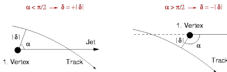
Slika 3.6: Skica rekonstrukcije parametra sudara miona. Izvor: [14]
