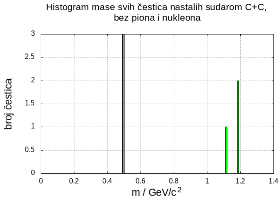
Slika 5: Histogram mase čestica nastalih sudarom C + C, bez piona i nukleona. Zaključujemo da, osim piona i nukleona, sudarom nastaje i mali broj kaona te \Lambda i \Sigma čestice.
