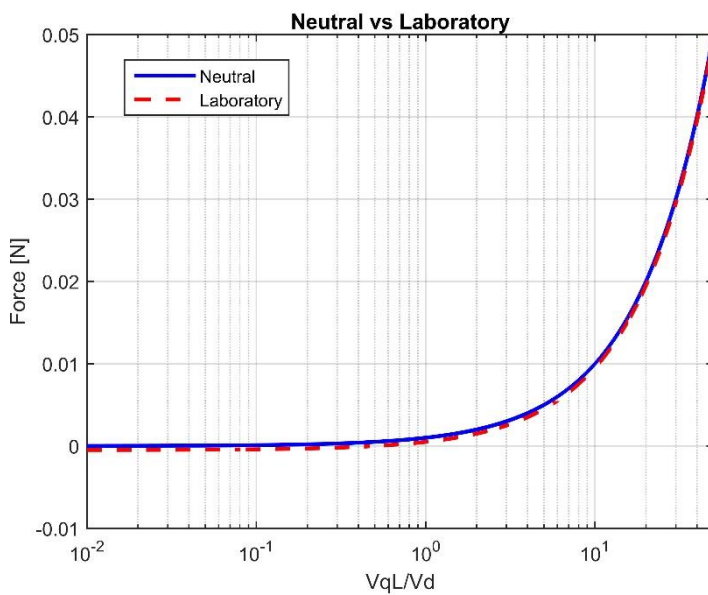
Slika 3.2 Usporedba sila u sustavu S_L a.) uvećano b.) umanjeno
