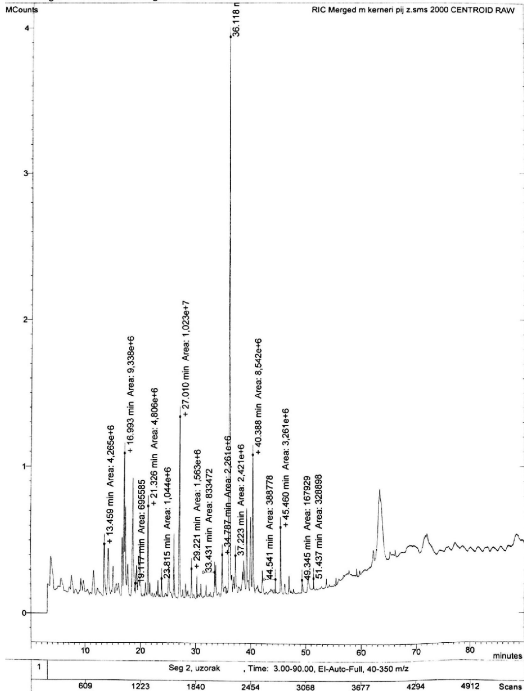
Slika 14.1: ukupne ionske struje za eterično ulje M. keneri (Izvor: Kremer i sur., 2013)
