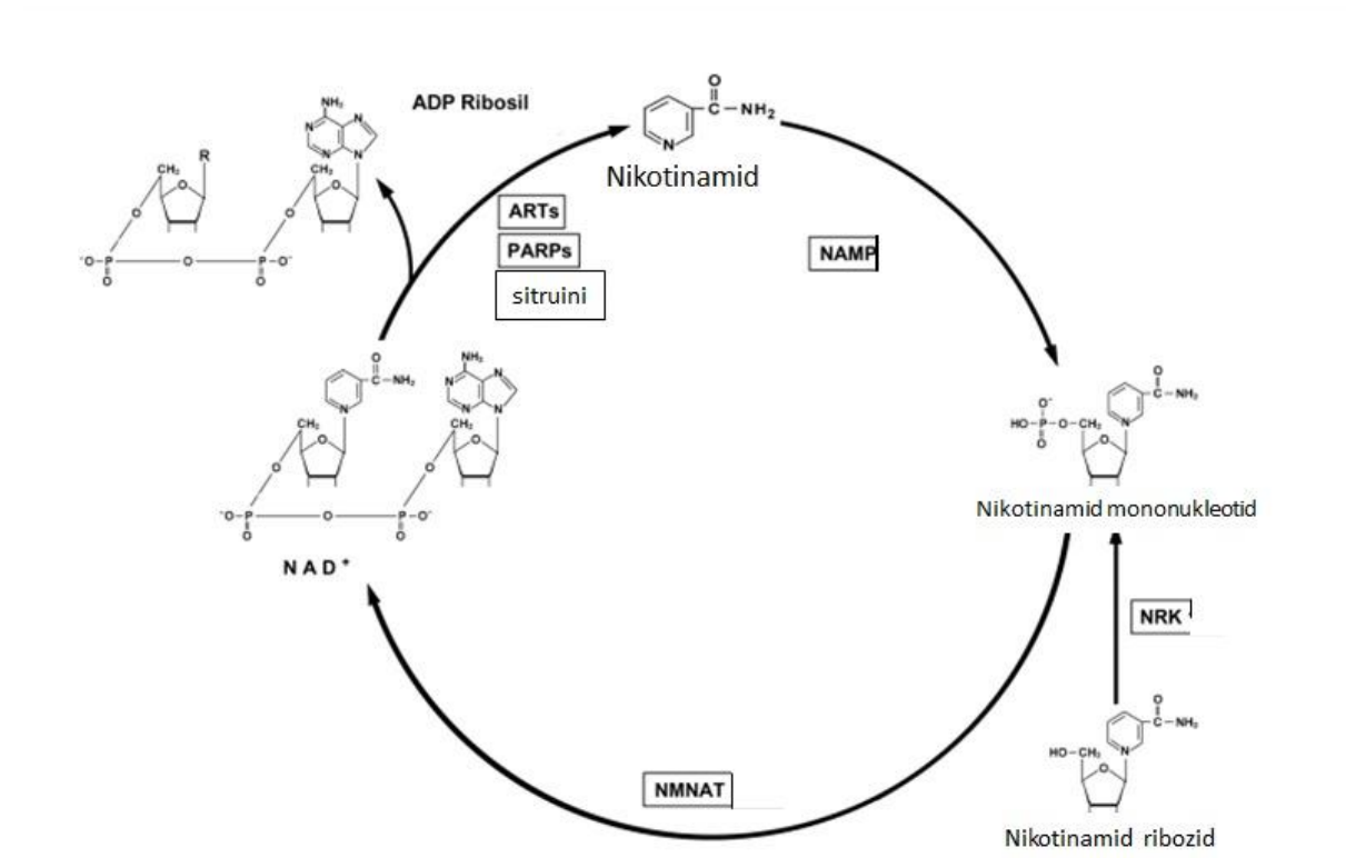
Slika 6. Recikliranje NAD + [1]
