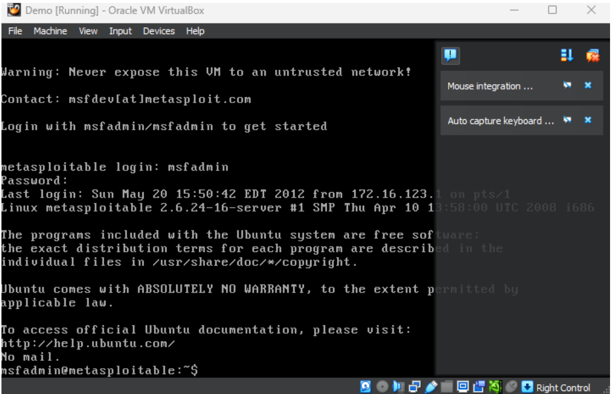
Slika 2.12 Metasploitable Linux
