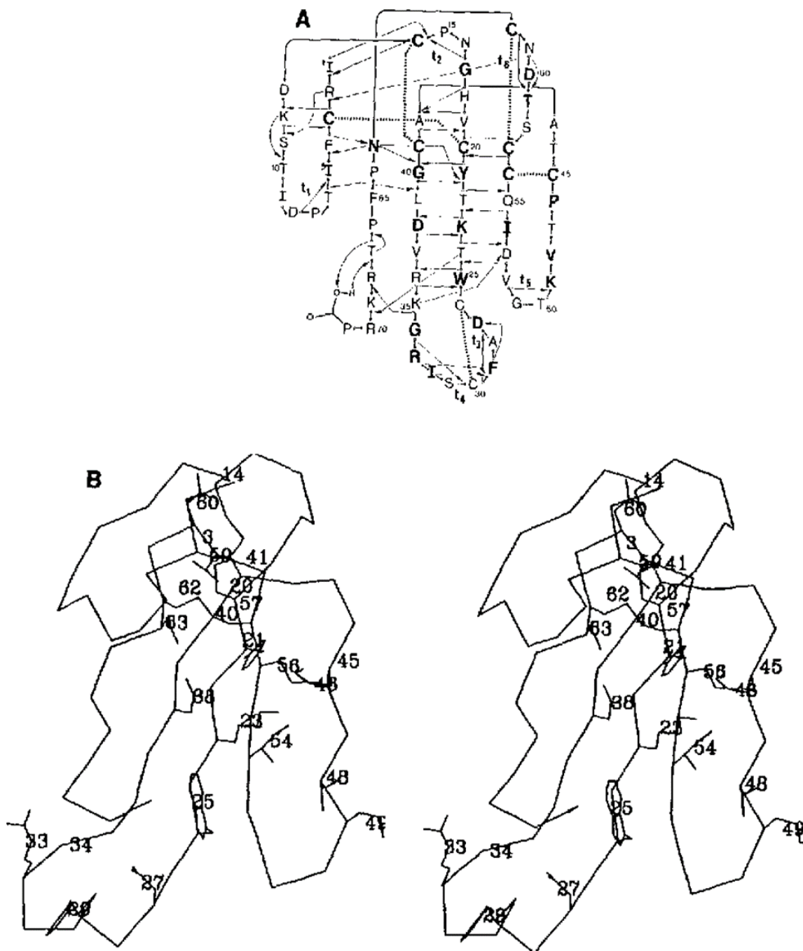
Slika 4. Prikazan je plan slijeda aminokiselina i unutarmolekularnih vodikovih veza \alpha -kobra toksina, a malim točkicama između cisteina prikazani su disulfidni mostovi (prikaz A). Prikaz B predstavlja stereo prikaz aminokiselina \alpha -kobra toksina (Betzel et al., 1991).
