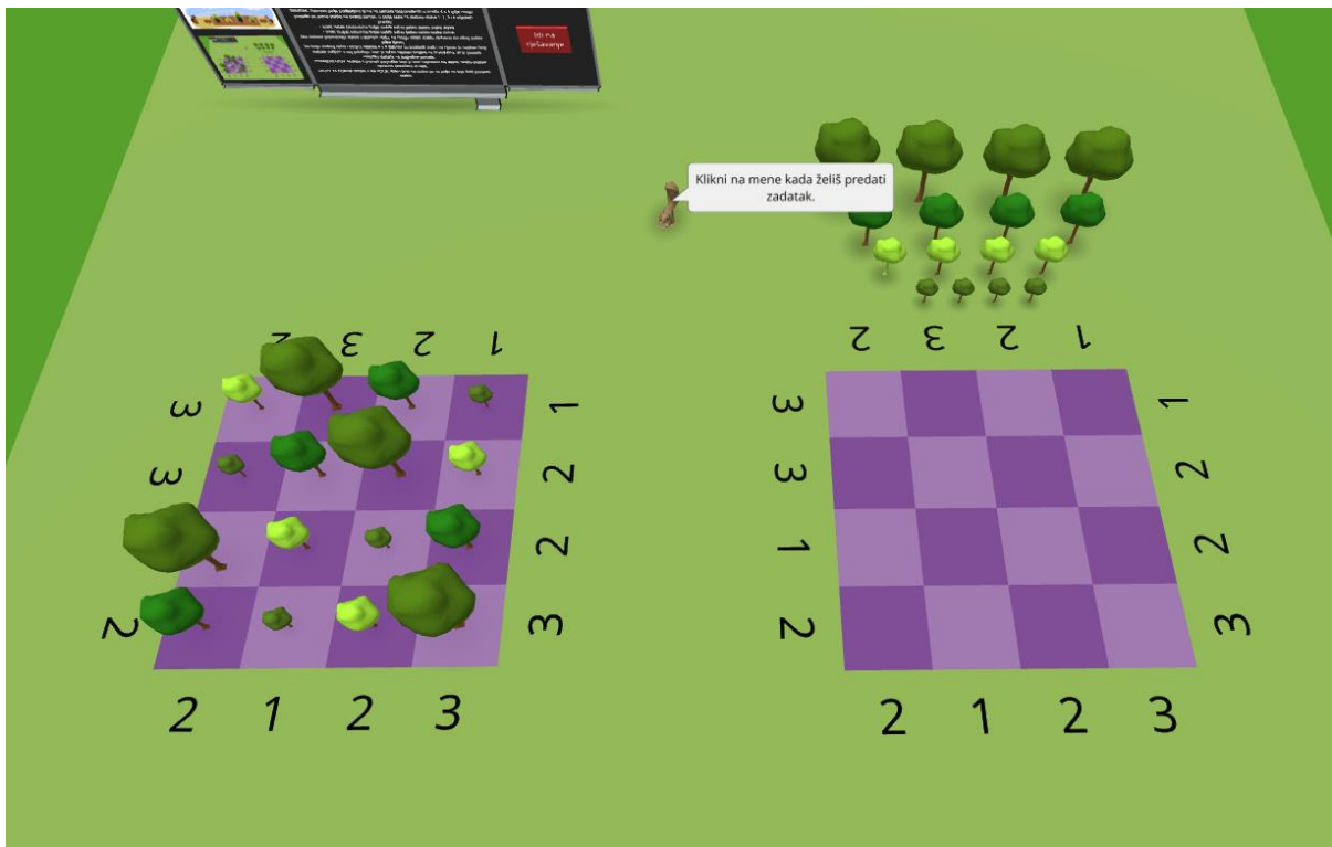
Slika 3.11 Sudoku stabla
