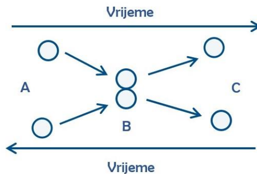
Slika 1. Shema sudara dviju kuglica i invarijantnosti na vrijeme. Položaj A predstavlja približavanje kuglica, položaj B sudar te položaj C ponovno udaljevanje. (prema ideji iz [1])
