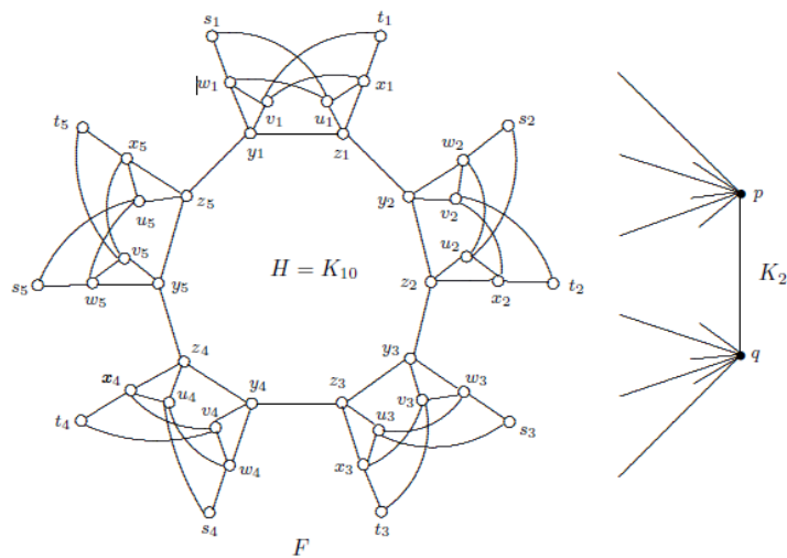
Slika 2.7: Bauer-Broersma-Veldmanov graf
