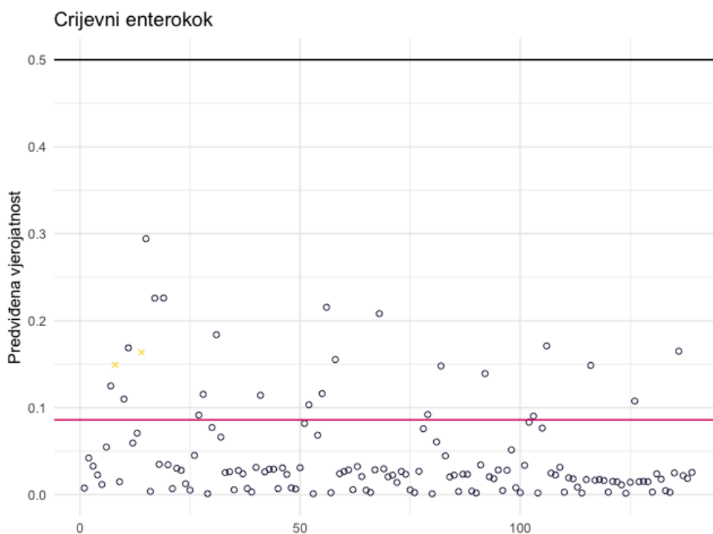
Slika 3.4: Predviđene vjerojatnosti za onečišćenje crijevnim enterokokijem
